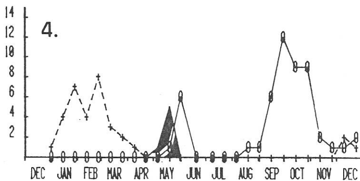
Fig. 2-4. Seizoenaal activiteitspatroon bij Carabidae van een bosbiotoop : Notiophilus biguttatus (fig. 2), Stomis pumicatus (fig. 3), Nebria brevicollis (fig. 4) Symboliek : adults : —○— ; tenels : —■— ; larven : ---+---
