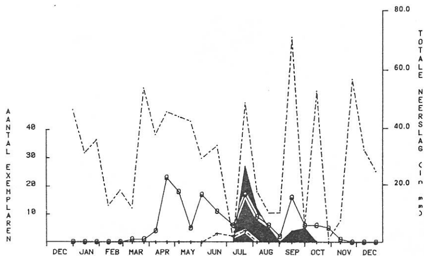
Fig. 8. Seizoenaal activiteitspatroon van Agonum assimile (adulten : ○; tenerals : ■; larven : ---) in relatie tot de totale neerslag (genoteerd te Brugge/Eeklo) tijdens de bemonsteringsperiode (symboliek : ····)
