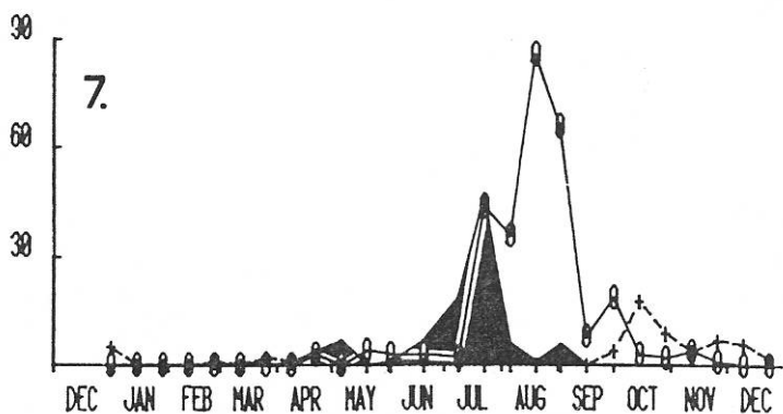
Fig. 5-7. Seizoenaal activiteitspatroon bij Carabidae van een bosbiotoop : Carabus purpurascens (fig. 5), Abax parallelepipedus (fig. 6), Calathus piceus (fig. 7) Symboliek : adulten : ○; tenerals : ■; larven : ---
